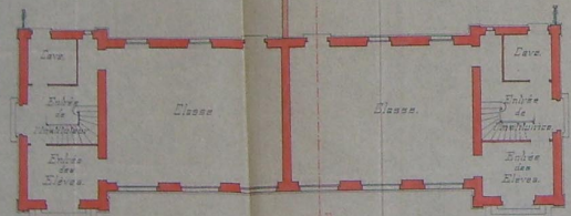
Plan du Rez-de-Chaussée.
